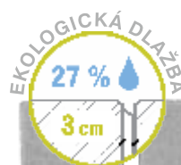
dolomite
