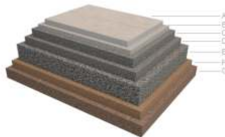
PRÍKLAD SKLADBY VRSTVIEV PRE VOZIDLÁ NAD 3,5 t
